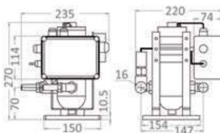
▲ Pompa alimentazione 50.237.50
