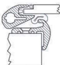
19.903.08 Braccetto di tenuta per portello boccaporto completo di supporti
