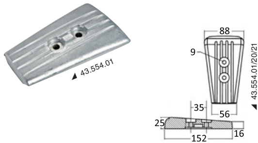
Anode legs SX/DPS
